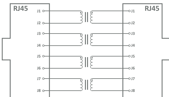
Netzwerkisolator MI 1005
